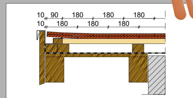
Lijevi završetak krova bez rubnog crijepa
