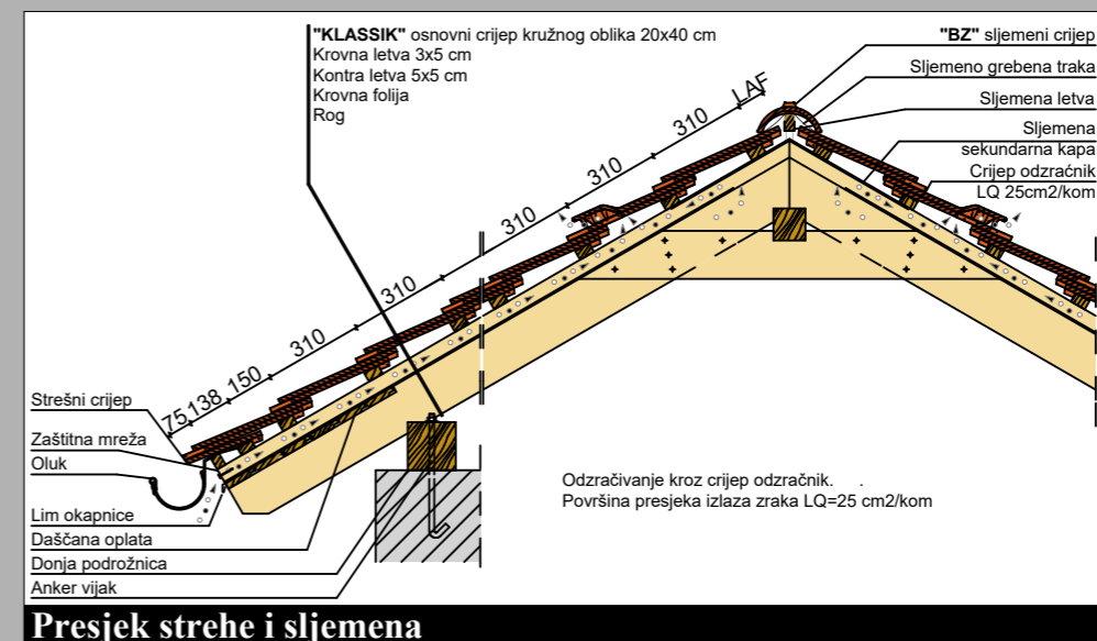
Presjek strehe i sljemena
