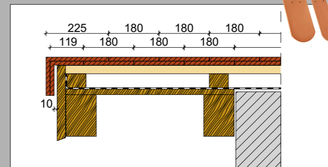
Završetak krova s lijevim rubnim crijepom
