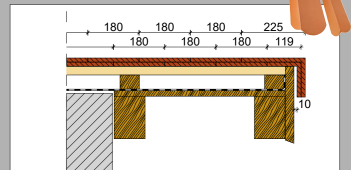
Završetak krova s desnim rubnim crijepom
