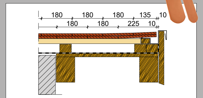
Desni završetak krova bez rubnog crijepa
